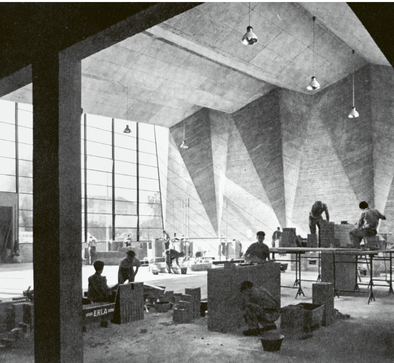
103 Maurerlehrhalle der Gewerbeschule Basel von Hermann Baur, erbaut 1958–1961.
