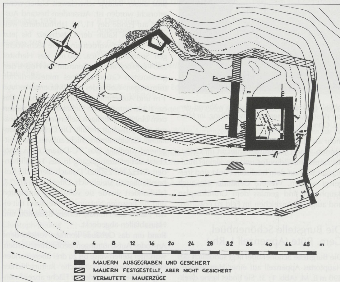
Abb. 2: Burgruine Clanx. Grundrissplan nach den Ausgrabungen von 1944/1949 (F. Knoll-Heitz).
