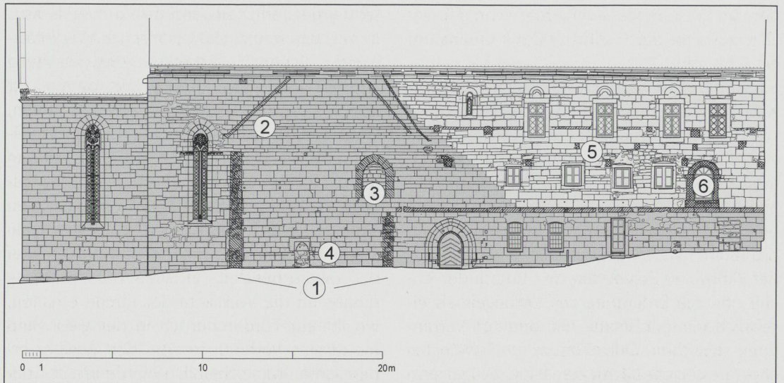
Abb. 3: Gnadental, Klosterkirche. Ansicht der Nordfassade (Ingenieurbüro Fischer/LDA). Vereinfacht wurden in Grautönen nur die beiden Haupt-Bauphasen der Kirche gekennzeichnet, ohne Baupausen, spätere Veränderungen, Fenstereinbrüche usw. zu berücksichtigen. Wesentliche Befunde sind schraffiert. 1 Anschluss des Ostflügels. Mit dem Mauerwerk verzahnt sind die Ostwand und das Erdgeschoss der Westwand, das Obergeschoss besaß eine Fachwerkkonstruktion; 2 Die Giebelkante an der Ostseite ist als massiver Anschlag beim Bau der Kirche vorbereitet worden, die Dachkante zum Klosterinneren wurde einfach gegen die Wand gesetzt; 3 Zugang zur Nonnenempore; 4 Sakristeitürchen; 5 ehemals doppelgeschossiger Kreuzgang, dessen Konstruktion vermutlich im 15. Jh. mit Einbau der unteren Konsolsteine nochmals verändert wurde; 6 nachträglich eingebrochener Emporenzugang.
