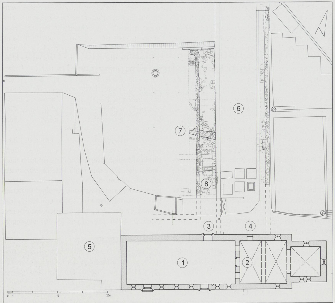
Abb. 1: Gnadental, Lageplan des ehemaligen Klosterareals (LDA): 1 Nonnenempore; 2 massive Trennwand zwischen Nonnenchor und östlichem Langhaus; 3 Kreuzgangportal; 4 Sakristeitürchen; 5 Äbtissinnenhaus; 6 Ostflügel, ergraben; 7 Wasserrinnen zur Trockenlegung des Geländes vor Baubeginn; 8 Kreuzgang mit aufgedeckten Grabplatten.
